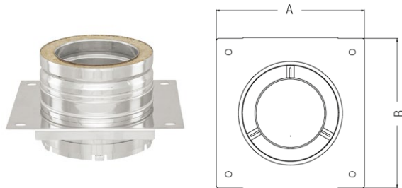
Zwischenstütze
