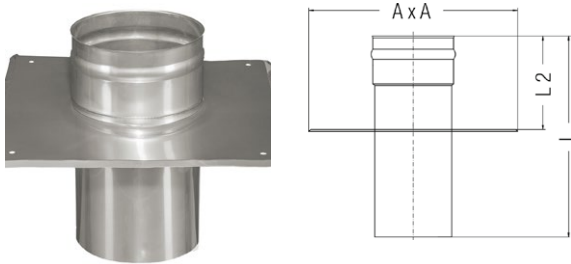
Schachtabdeckung, ohne Hinterlüftung
