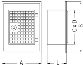
Reinigungstür mit Schiebestutzen und Lüftungsgitter
