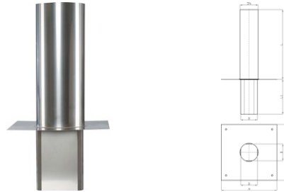
Schornsteinverlängerung, Einsteckende eckig
