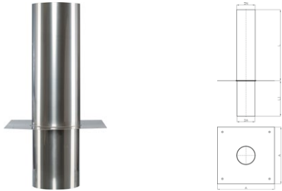
Schornsteinverlängerung, Einsteckende rund
