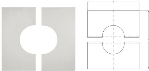
Abdeckblende
